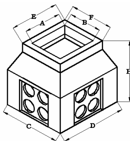
ARQUETA A1 H=105
