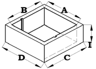
SUPLEMENTO ARQUETA
