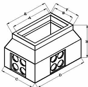
ARQUETA MEDIA TENSION A2 H=105
