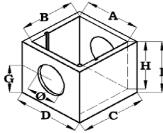
ARQUETA SANEAMIENTO
